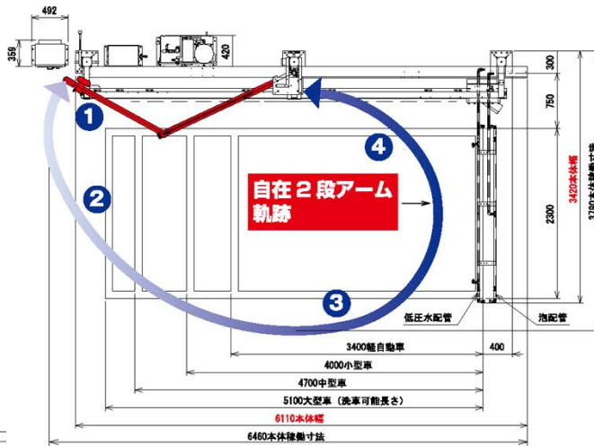
水と泡が出るブームは水平の一本のみとし、吹き出しノズルの角度を吟味して、前後横も洗えるようにして垂直の可動ノズルを廃止。ブームが移動する速度は自在に変えられます。
